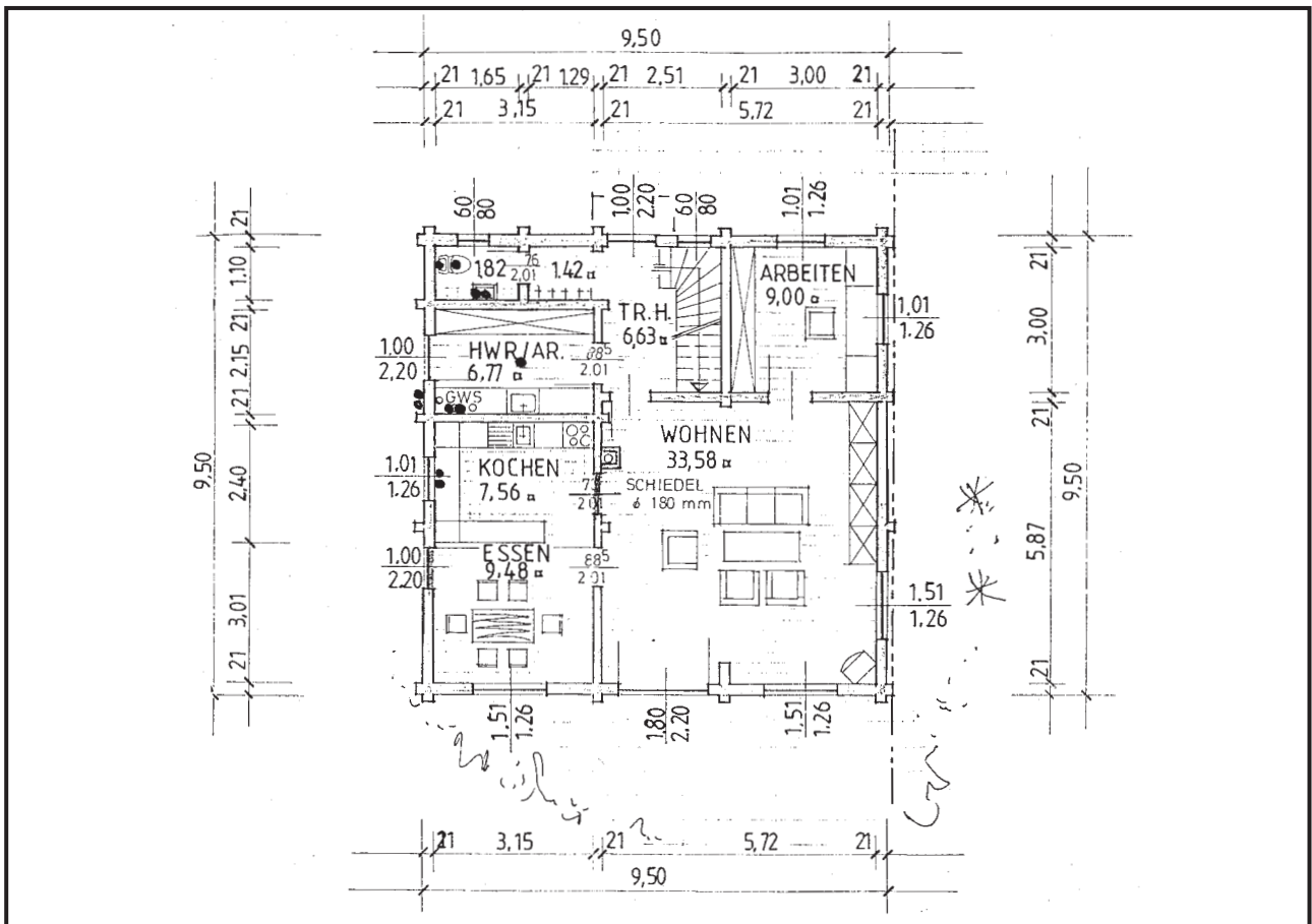
ERDGESCHOSS
