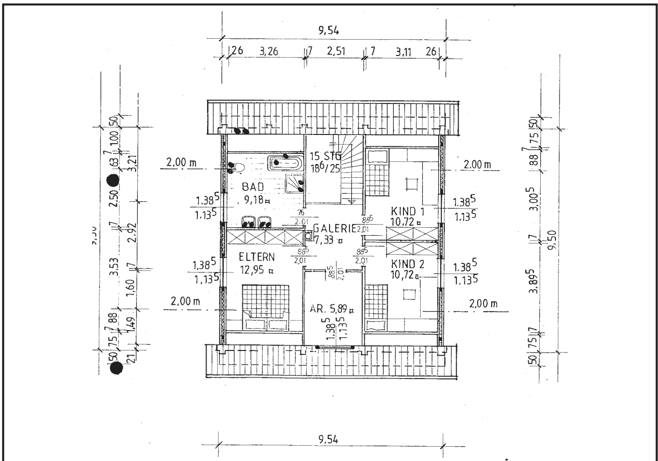
DACHGESCHOSS
