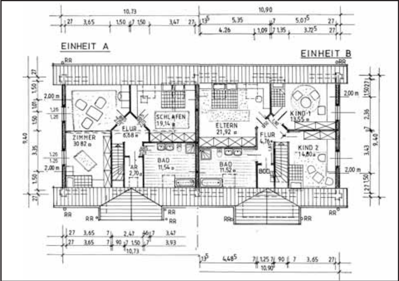
DACHGESCHOSS
