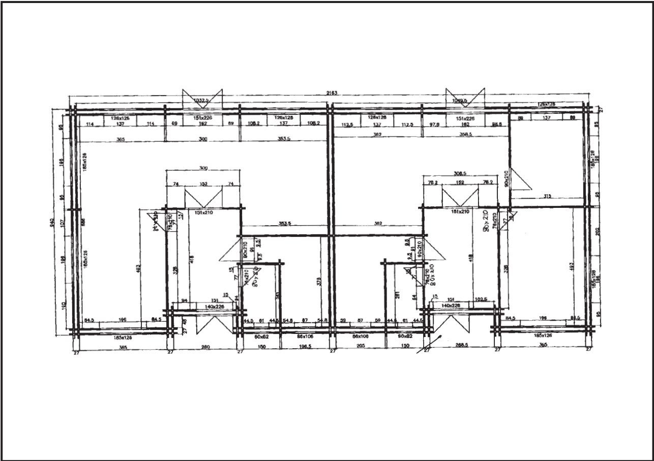
ERDGESCHOSS
